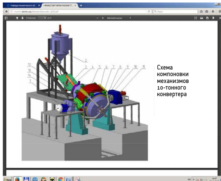
3D-модель конвертера
